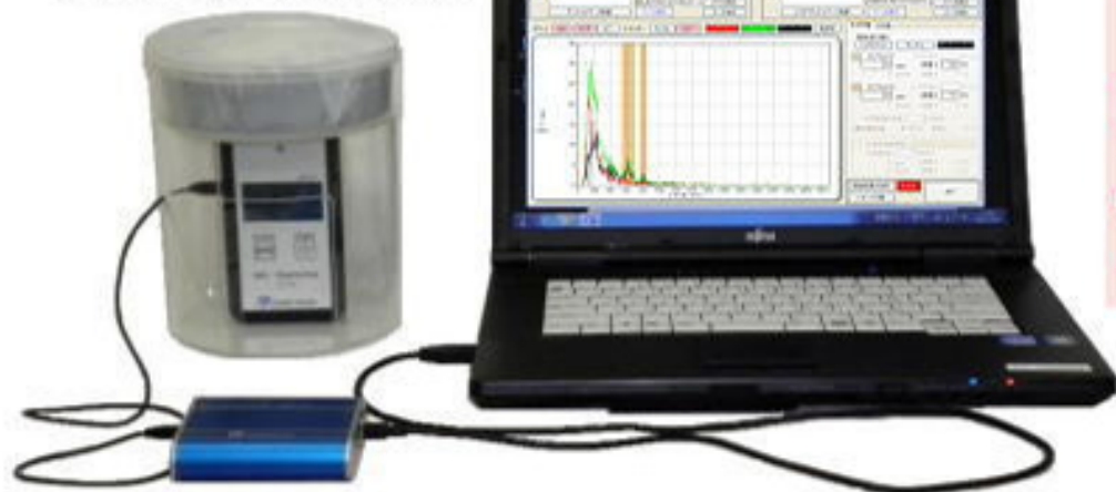
A2702型 Mr. Gamma MCA
